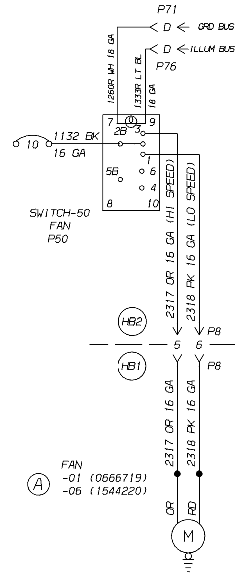
FEA 30026-01,06 AUX FAN UPPER RIGHT
