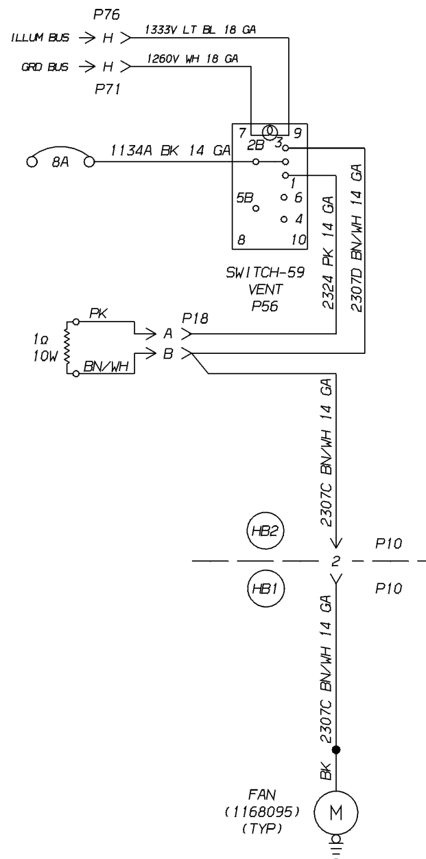
EXHAUST FAN 2 SPEED - QTY 1
