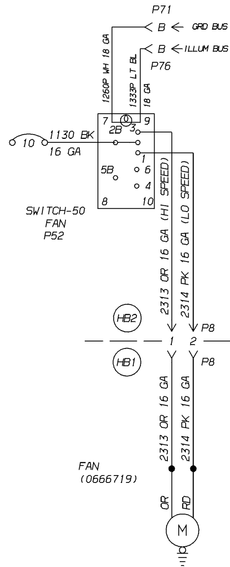
FEA 30026-03 AUX FAN UPPER CENTER
