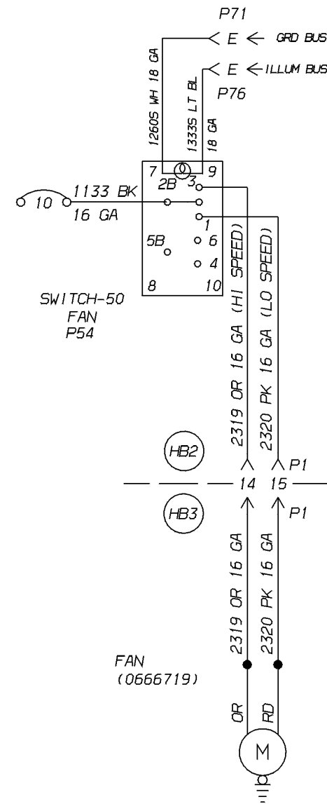
FEA 30026-05 AUX FAN LOWER RIGHT
