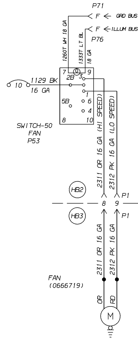
FEA 30026-04 AUX FAN LOWER CENTER W/S
