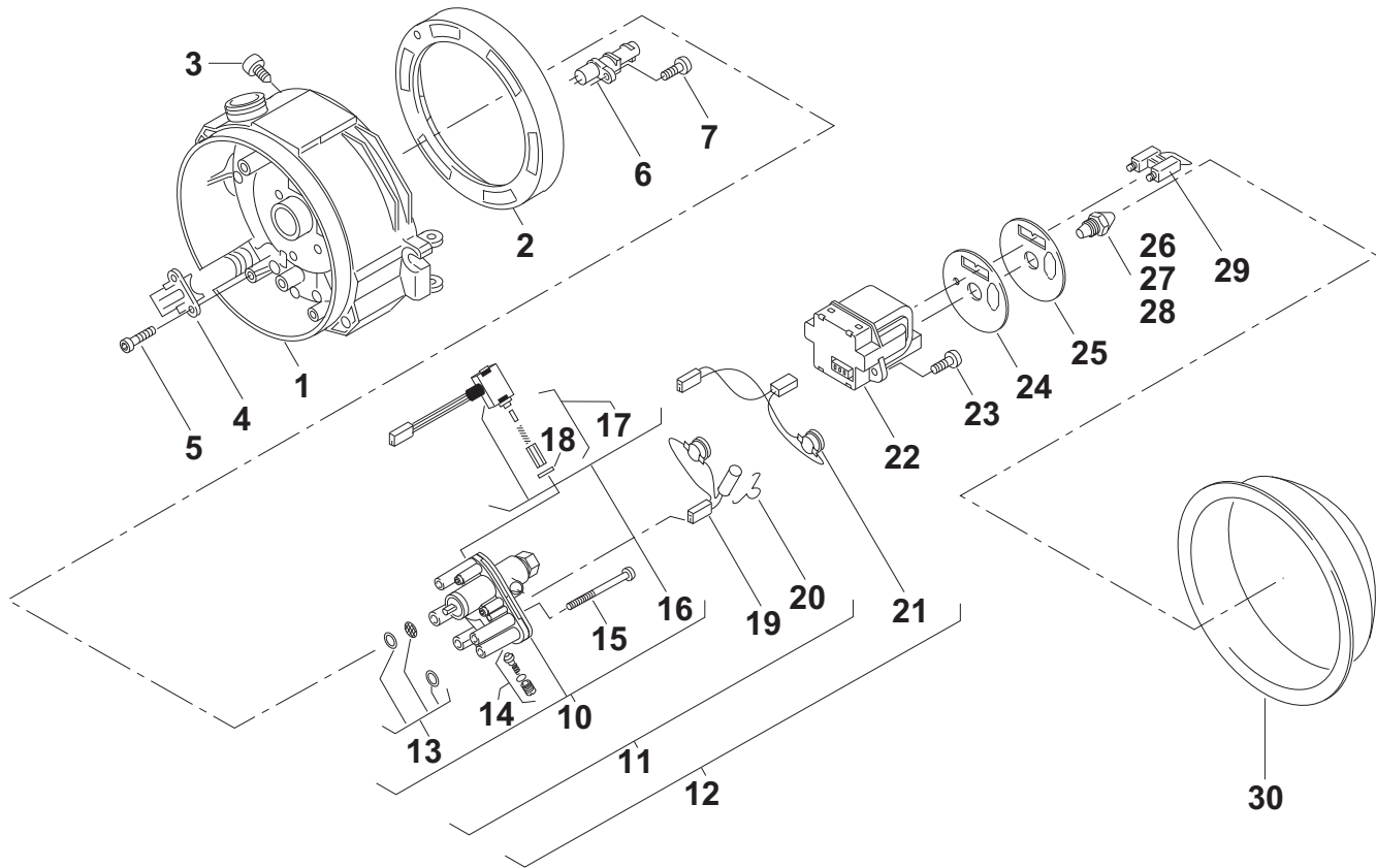
Thermo 230 / 300 / 350 - fig. 2
