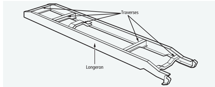
FIGURE 18 | Châssis (longerons et traverses)
