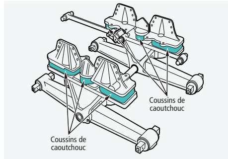
FIGURE 51 | Suspension avec coussins de caoutchouc
