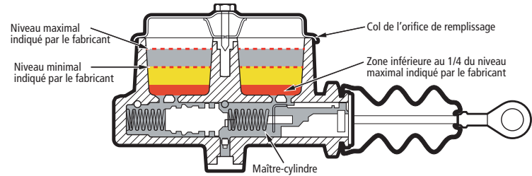
FIGURE 58 | Réservoir du maître-cylindre avec indicateurs du fabricant
