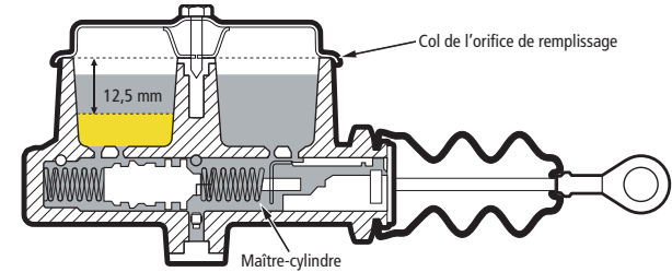
FIGURE 59 | Réservoir du maître-cylindre sans indicateurs du fabricant
