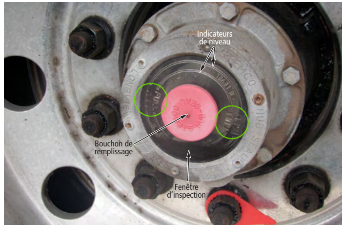
FIGURE 46 | Fenêtre d'inspection d'un moyeu de roue
